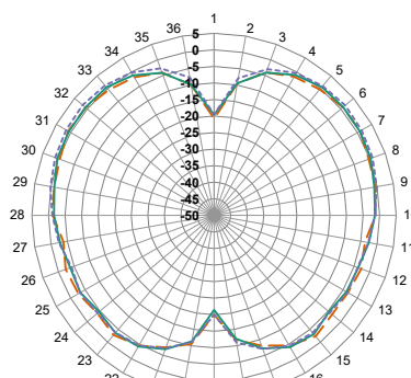
YZ-Plane Gain
