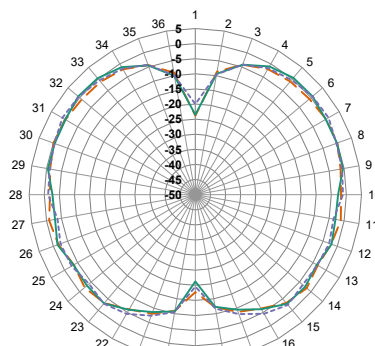
YZ-Plane Gain
